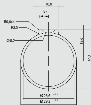
SEZIONE FUSTO BARREL SECTION
